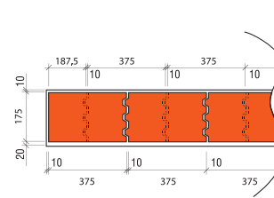
TD 175 PD AKUSTIK
