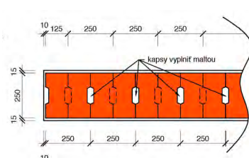
TD 250 PD AKUSTIK ZK
